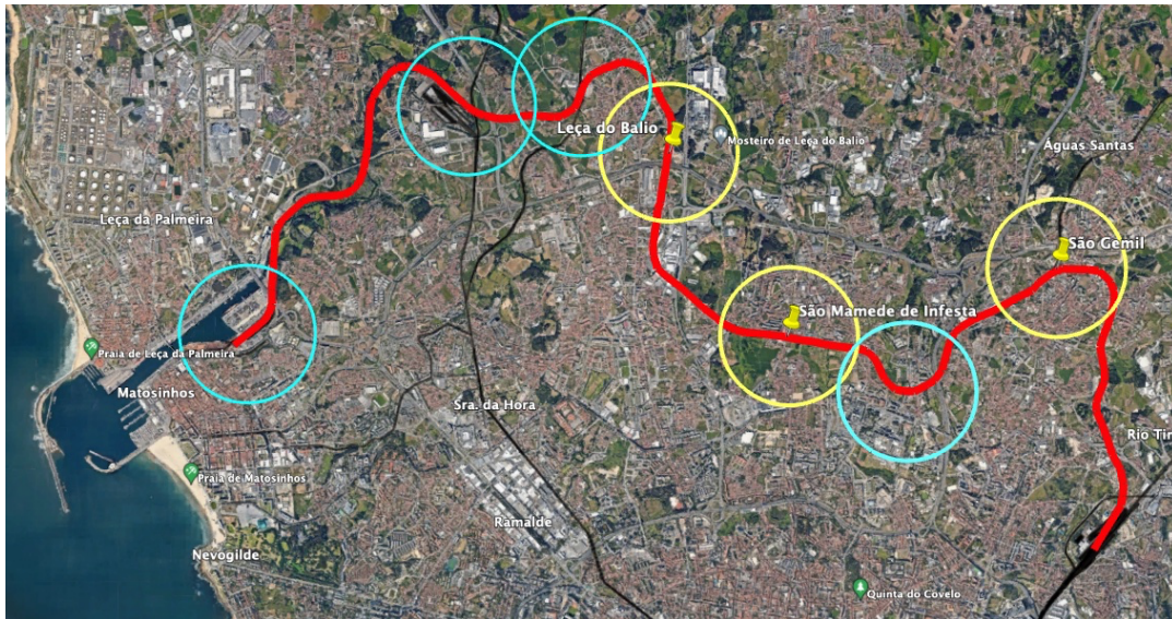
Figura 22. Traçado da Linha de Leixões com raios de 750 m, correspondentes a uma distância a pé de aproximadamente 10 minutos, representados a partir das estações existentes (amarelo) e propostas (azul-claro). As localizações propostas para novas paragens correspondem aos pontos em que a Linha de Leixões intersecta ou se aproxima da rede do Metro do Porto.
