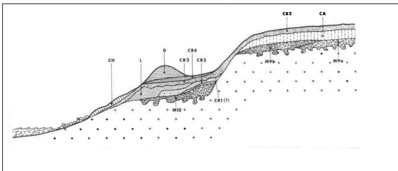
Fig. 1 – Corte geológico esquemático-interpretativo (sintético) da disposição dos depósitos estratigráfico do Quaternário do Litoral do Minho, segundo Meireles (1992).
